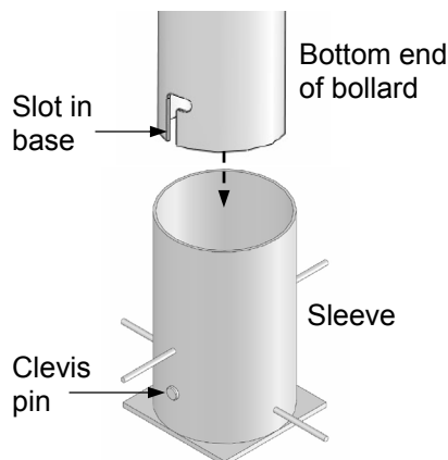
FIG. 5A: Install bollard
